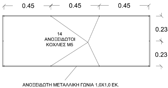
ΠΛΑΙΣΙΟ ΣΤΗΡΙΞΗΣ ΕΝΗΜΕΡΩΤΙΚΗΣ ΠΙΝΑΚΙΔΑΣ ΕΠΙ ΣΚΥΡΟΔΕΜΑΤΟΣ
